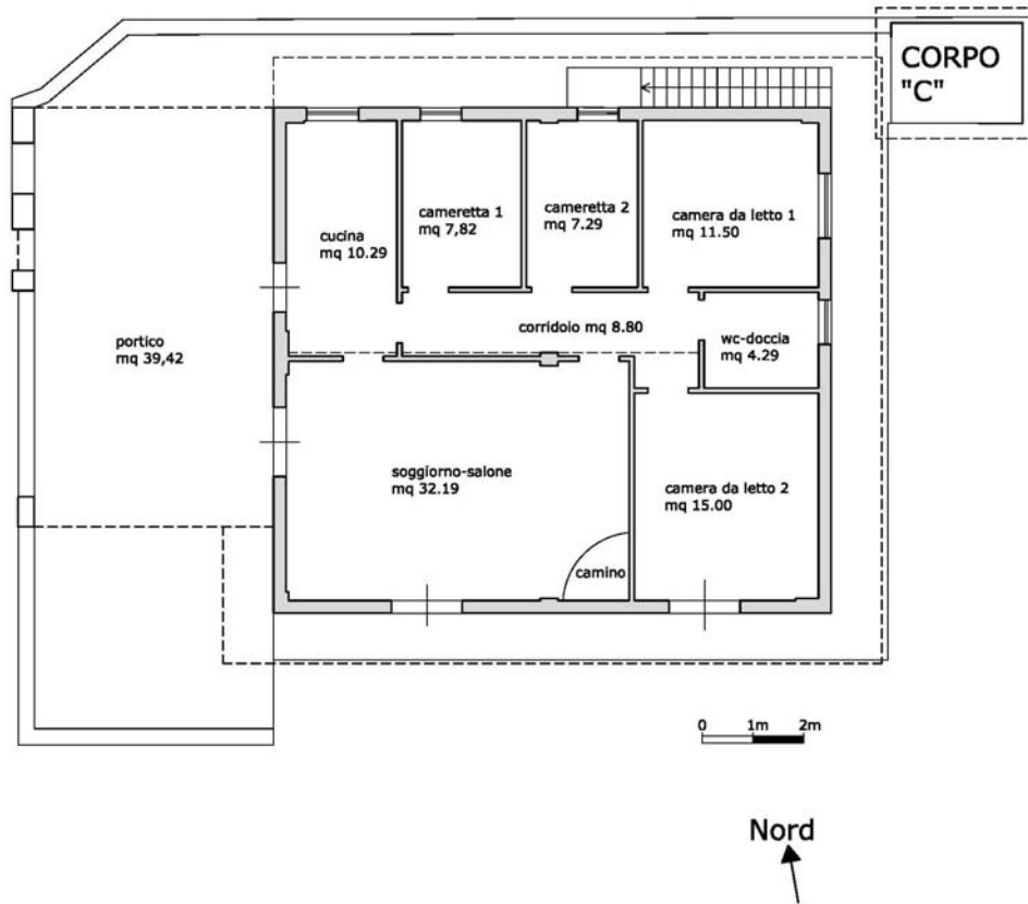
Planimetria di rilievo dello stato di fatto corpo "A" (All. 18a)
