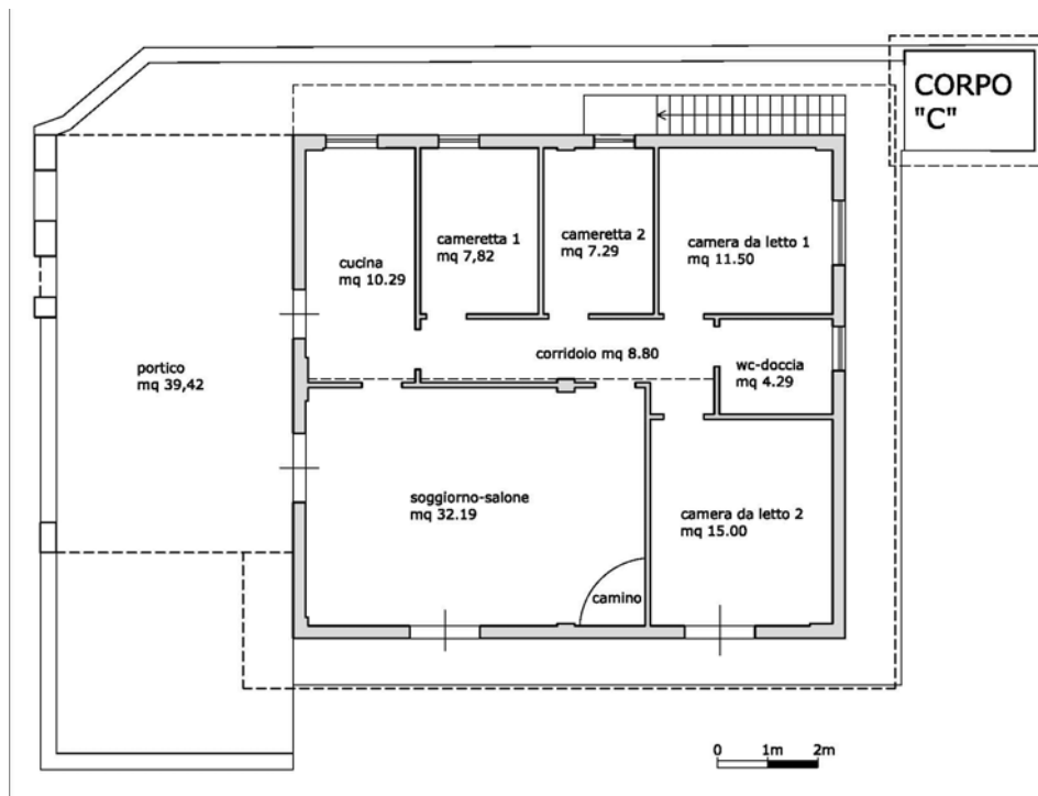
Planimetria di rilievo attuale
